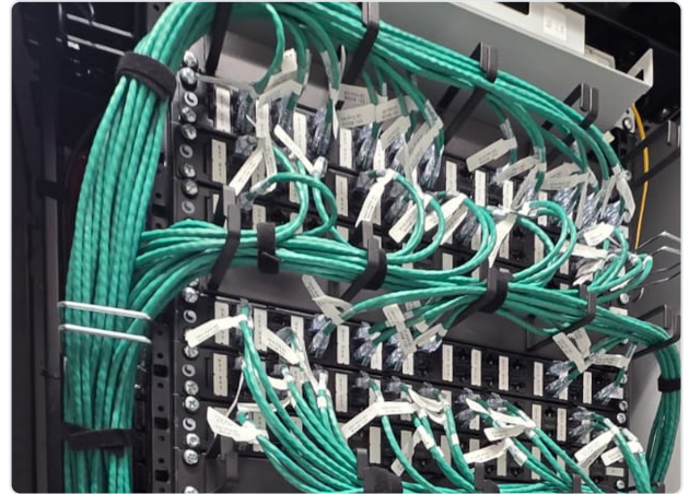
Camera server — patchare etichetată la nivel de port, pe management de cabluri.
