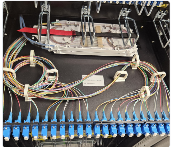
Terminații de fibră optică OS2 — panou LIU cu 24 de adaptoare LC/UPC și tavă de splice.
